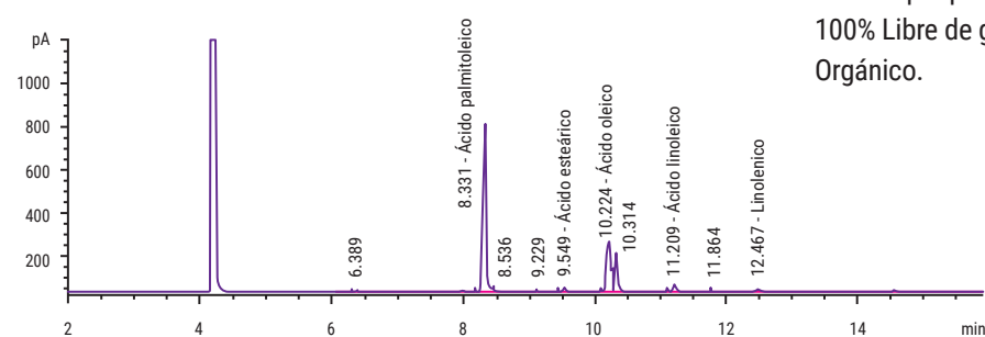
Gráfica 1. Perfil cromatográfico mediante HPLC del contenido en omegas 3,6,7 y 9 de las bayas del espiño amarillo.
